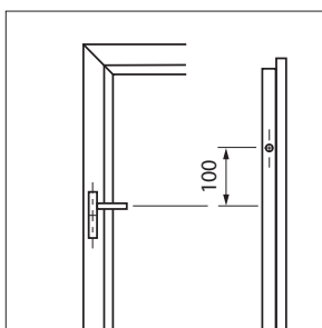
dictator deurveer opdek bovenzijde deur
