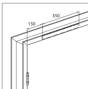
deurdranger voorziening voor brandwerende kozijnen zonder bovenlicht
