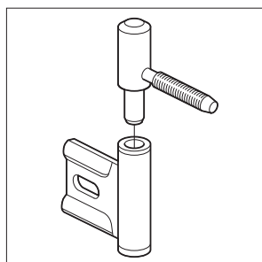
MonoPlus paumelle voor MonoPlus montagekozijnen, in opdekuitvoering, verzinkt
