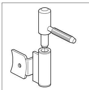
Z-paumelle voor Solid inmetSELkozijnen, in opdekuitvoering, verzinkt
