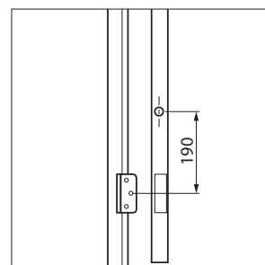
dictator deurveer stomp onderzijde deur
