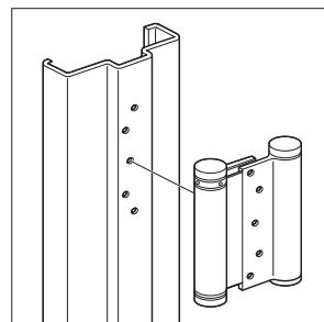
bommerscharnier t.b.v. doordraaideuren
