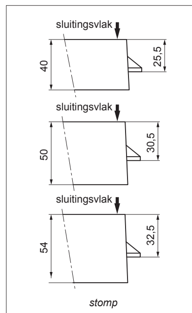
maatvoering schoot
