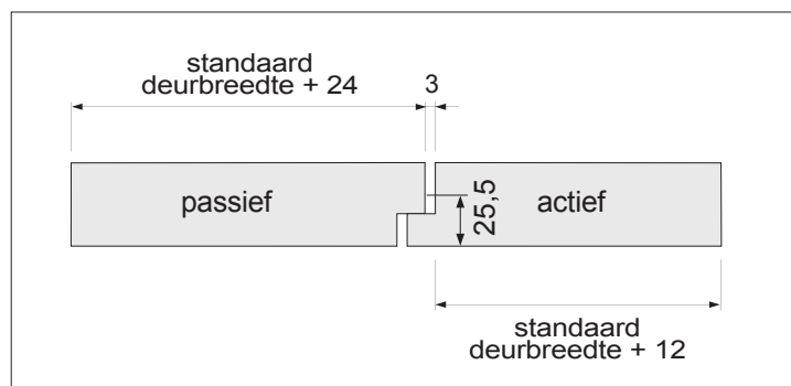
horizontale doorsnede stomp dubbeldeursuitvoering, spooling-contraspooling
