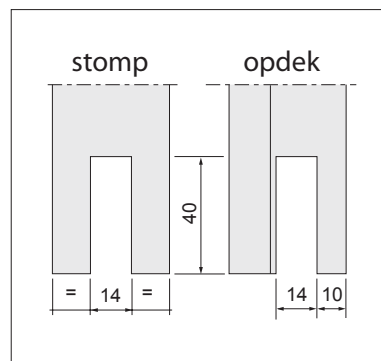
groef onderkant deur t.b.v. valdorpel
