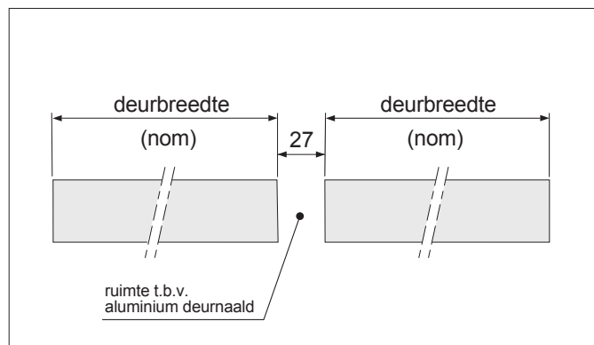
horizontale doorsnede stomp dubbeldeursuitvoering met Alprokon P-deurnaald
