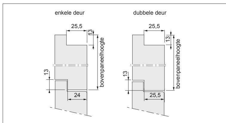
verticale doorsnede bovenpaneel, opdek "recht"
