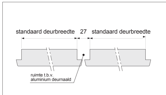
horizontale doorsnede opdek dubbeldeursuitvoering met Alprokon deurnaald type 27
