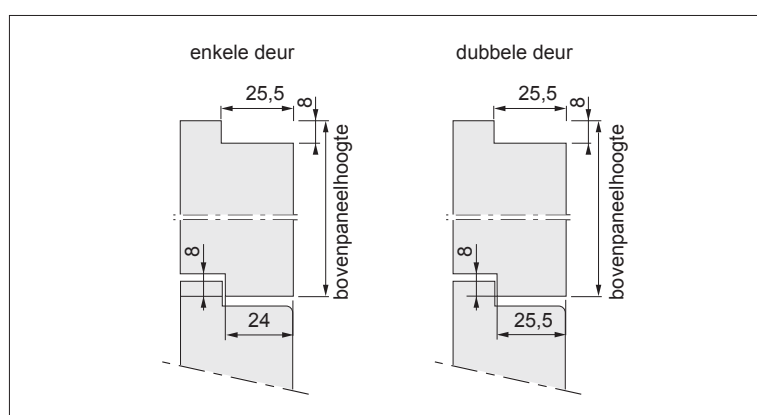
verticale doorsnede bovenpaneel, opdek "schuin"
