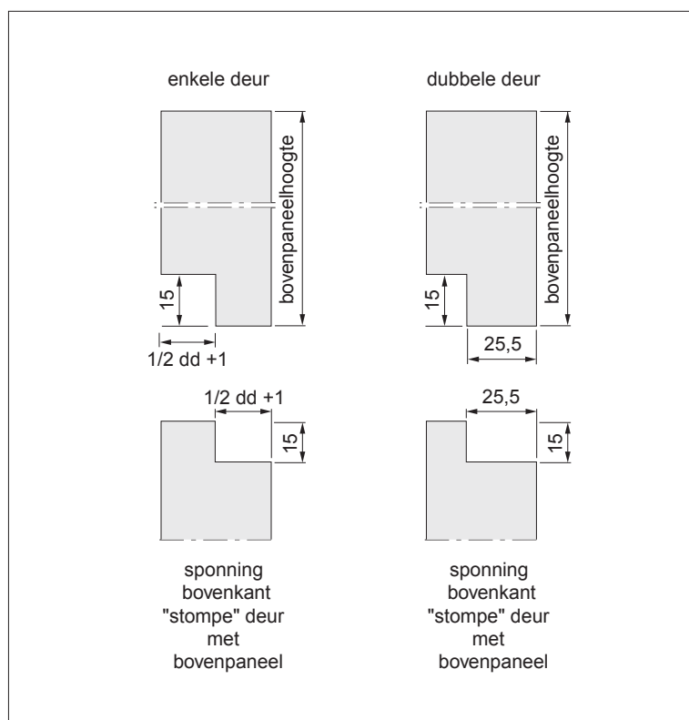
verticale doorsnede bovenpaneel
