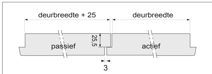
horizontale doorsnede opdek dubbeldeursuitvoering, spooling-contraspooling
