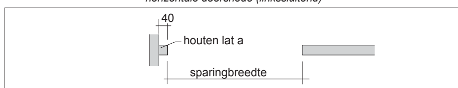
horizontale doorsnede, met haakse wandaansluiting (linkssluitend)
