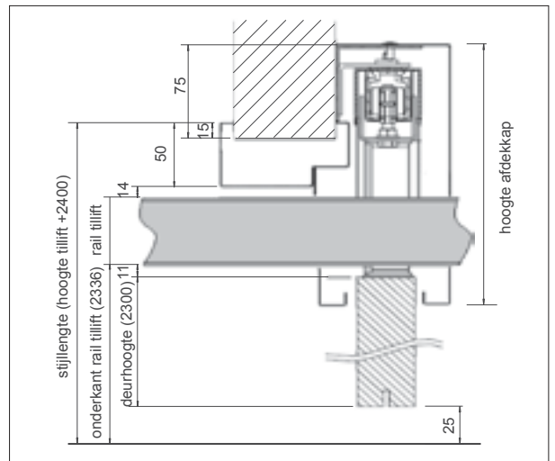
verticale doorsnede SVW 1 t.b.v. tillift
