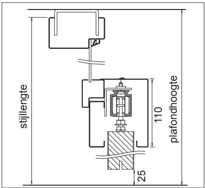
verticale doorsnede SVW2
