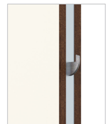
Serrure 3 points avec 2 pènes crochets
