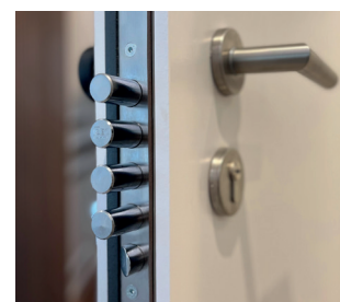
5 van de 8 sluitpunten van de Steel Secure deur
